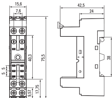
Рис. 2 Габаритные размеры PM Slim 22/2 EKF AVERES
