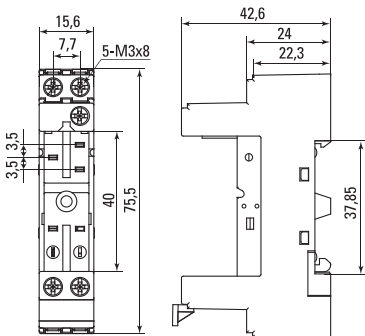
Рис. 1 Габаритные размеры PM Slim 25/1 EKF AVERES
