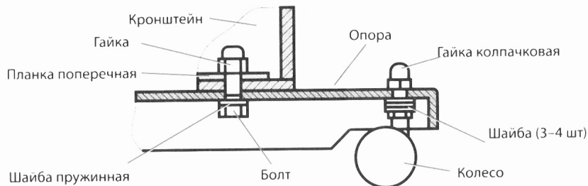
Рис. 3в. Крепление опоры с колёсами
