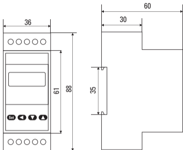
Рис. 2 Габаритные размеры
