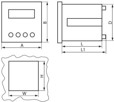
Рис. 2 Габаритные размеры
