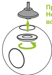
5.4. Собрать светильник.
