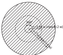
Рисунок 2. Зоны обнаружения датчиков движения ДДМ-01
