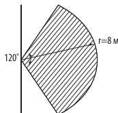
Рисунок 2. Зоны обнаружения датчиков движения ДДМ-01
