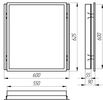
Рисунок 5 — Габаритные размеры светильников серии Экофон.
