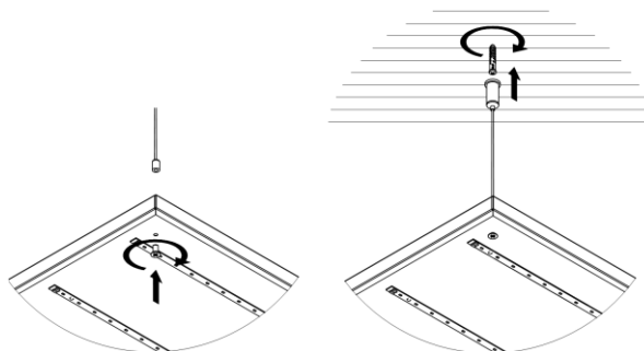
Рисунок 11 — Подвесной монтаж.
