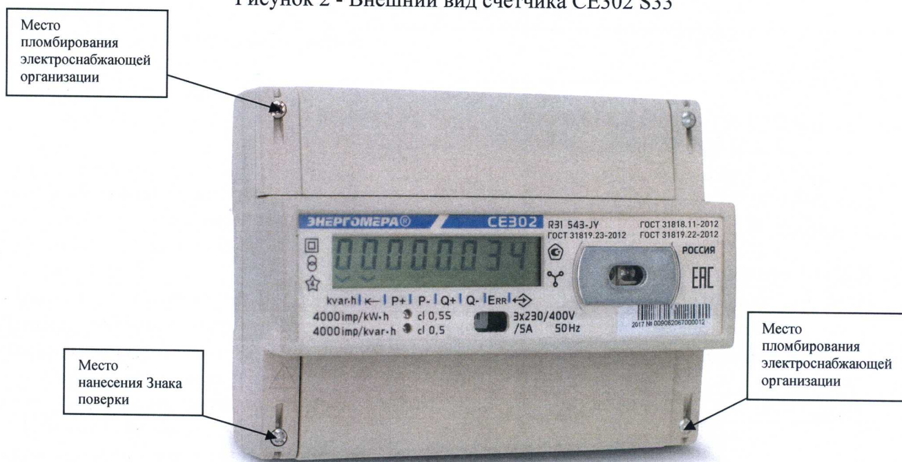
Рисунок 3 - Внешний вид счетчика CE302 R31
