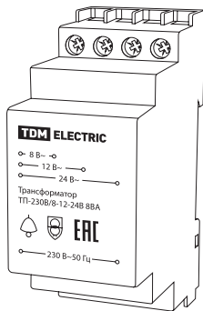
Рисунок 1. Внешний вид трансформатора ТП-230B/8-12-24B
