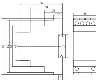
Рисунок 2. Габаритные и установочные размеры трансформаторов, мм
