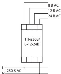
Рисунок 3. Схема подключения трансформатора ТП-230В/8-12-24В к сети
